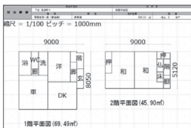
○家屋平面図
